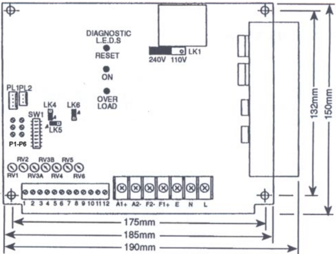
Рис. 1 Общий вид привода SHEETAH SM
